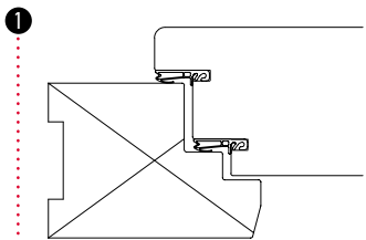
Standardausführung Stock und Flügel ca. 70 mm stark; innen und außen überfäلت
