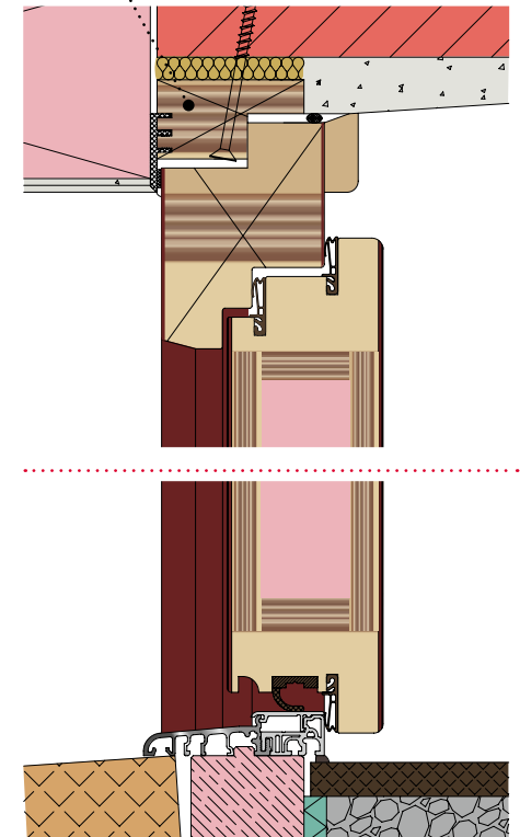
Einbau mit Blindstock
