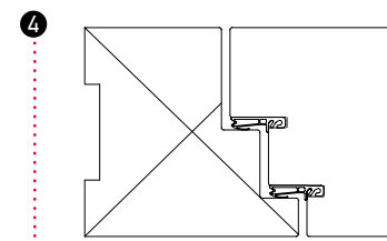
Ausführung: IBAB Stock und Flügel ca. 100 mm stark; innen und außen bündig
