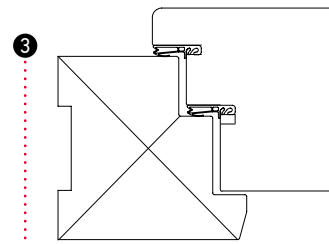
Ausführung: Standard 100 Stock und Flügel ca. 100 mm stark; innen und außen überfäلت
