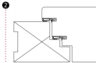
Ausführung: ISAB Stock ca. 70 mm / Flügel ca. 100 mm stark; innen standard, außen bündig
