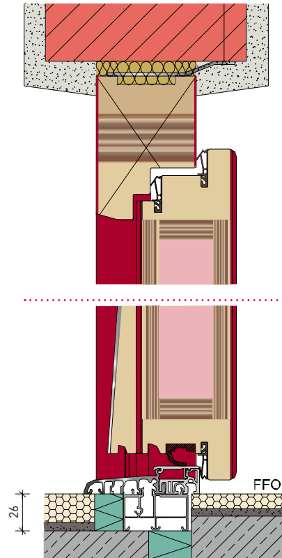
Einbau ohne Blindstock
